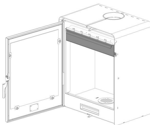
Figura nº5 - Accesorio de ayuda para casos de revoques de humos causados por una instalación deficiente
