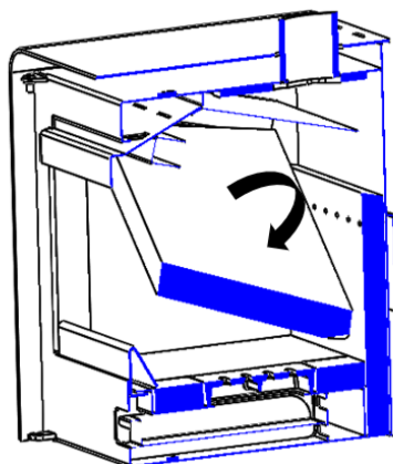
Figura n°9 - Extracción de los deflectores de vermiculita
