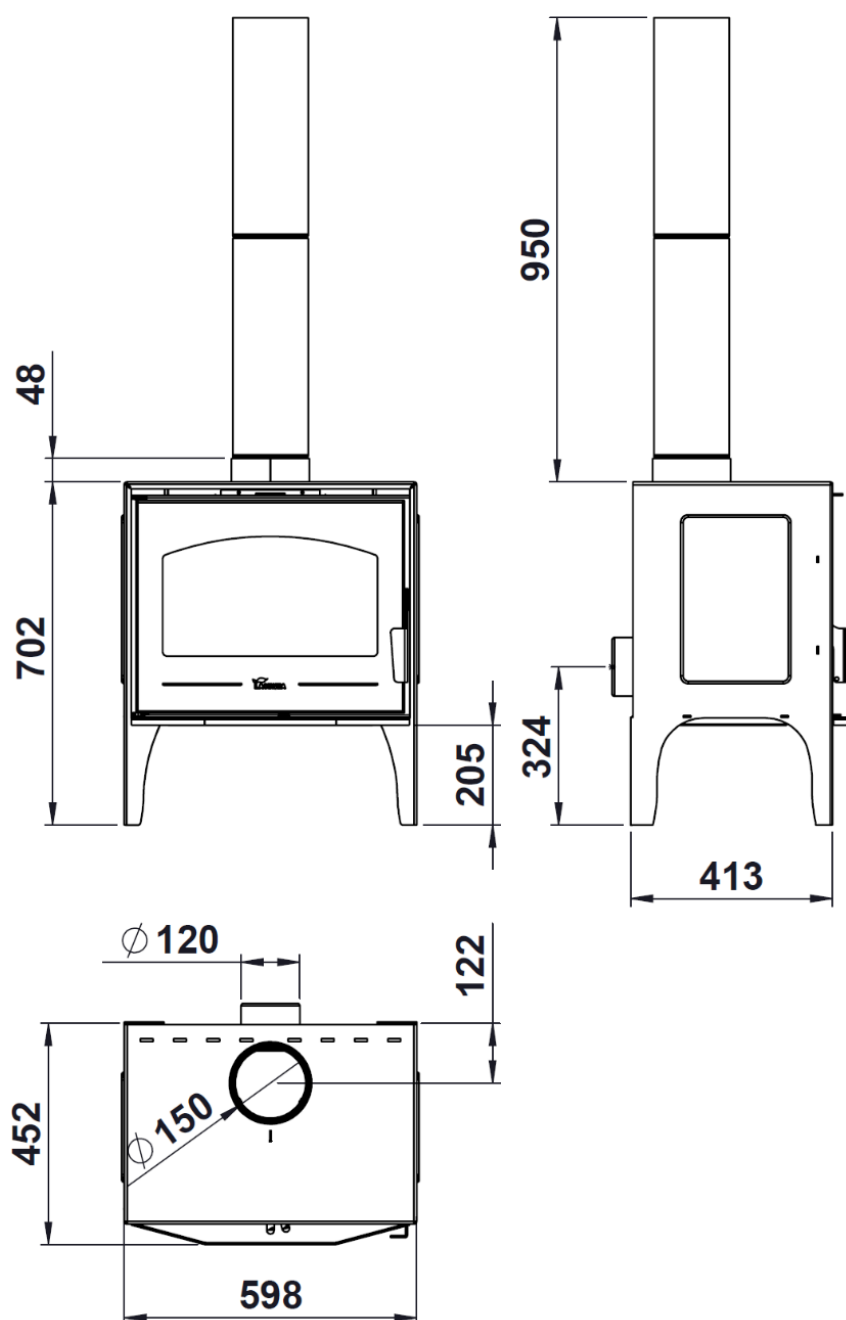
Figura n°1 - Dimensiones en mm de la CALPE STAR
