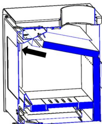
Figura n°8 - Primer movimiento para liberar el refuerzo
