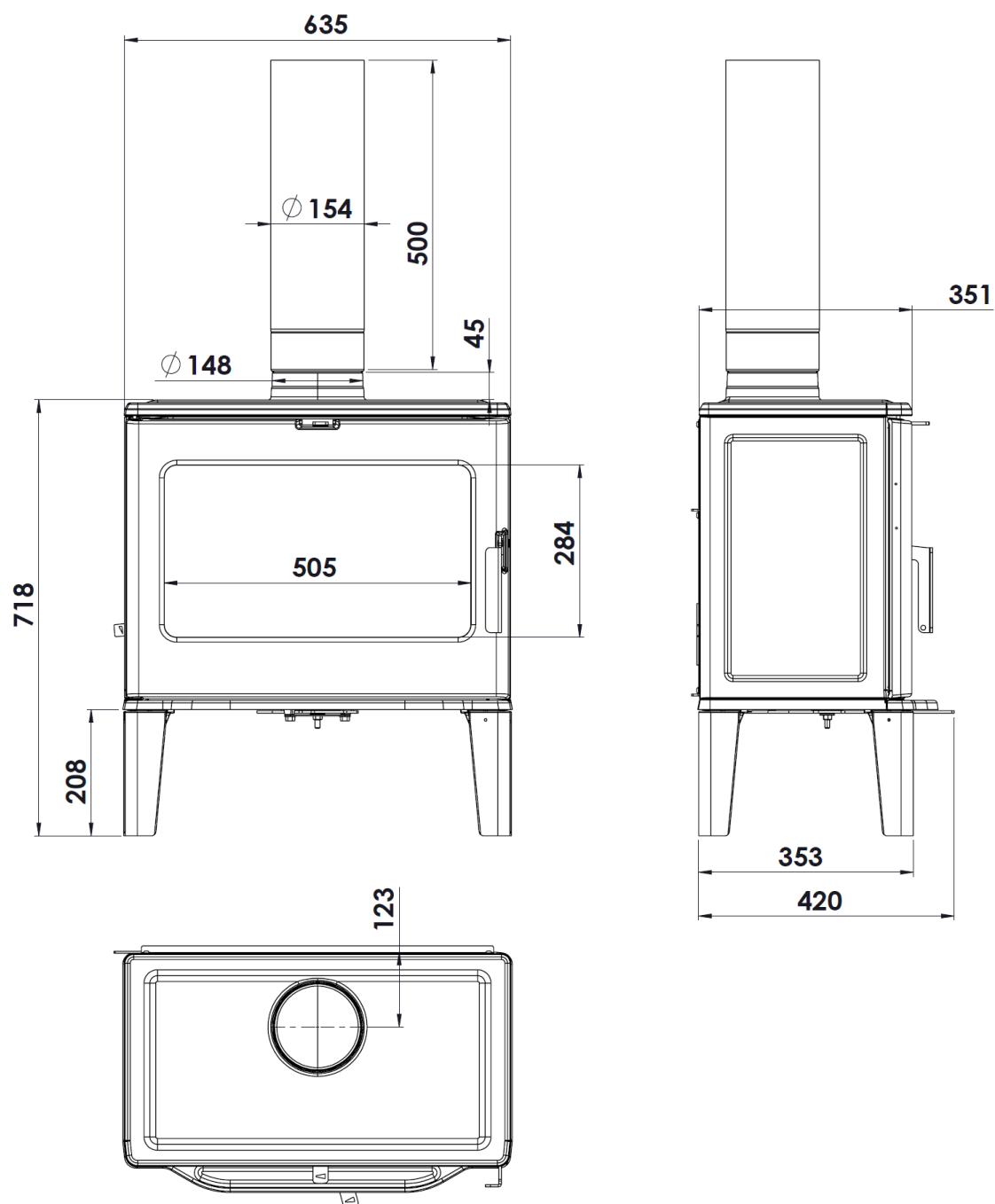
Figura nº1 - Dimensiones en mm del aparato Bidart
