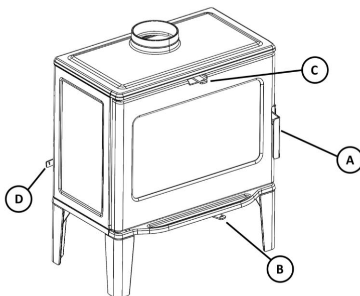
Figura nº9 - Elementos de funcionamiento del aparato
