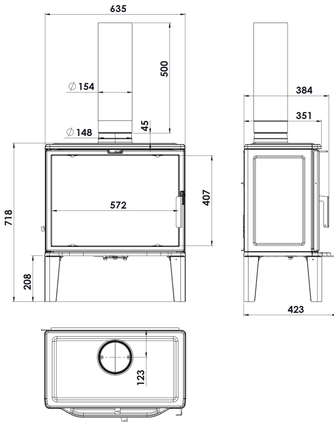
Figura nº1 - Dimensiones en mm del aparato Biarritz
