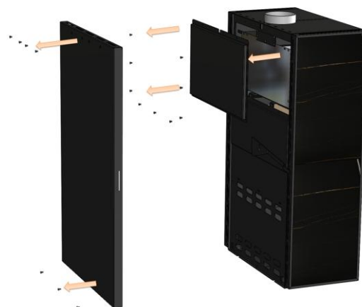
Figura n°17 - Desmontaje tapa trasera BERGEN
