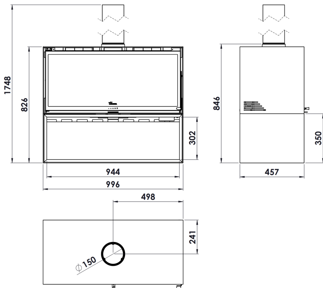
Figura nº5 - Dimensiones en mm del aparato BAIONA 1000
