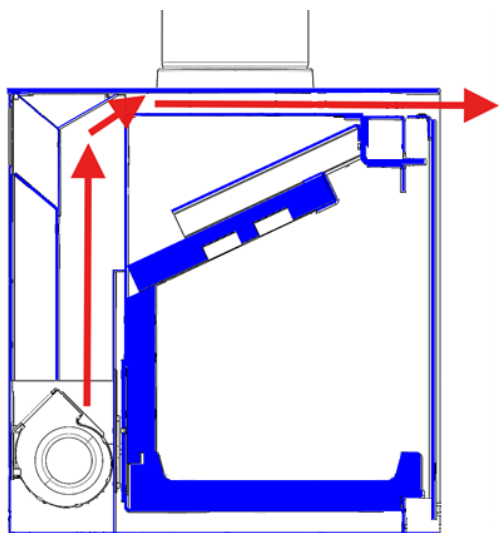
Figura nº16 - Recorrido del aire caliente sin canalizaciones
