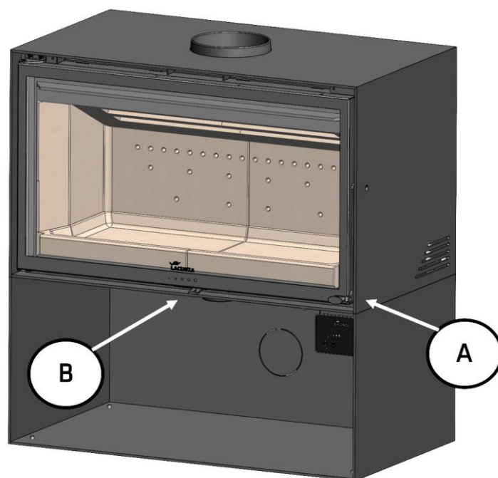
Figura n°24 - Elementos de funcionamiento del aparato
