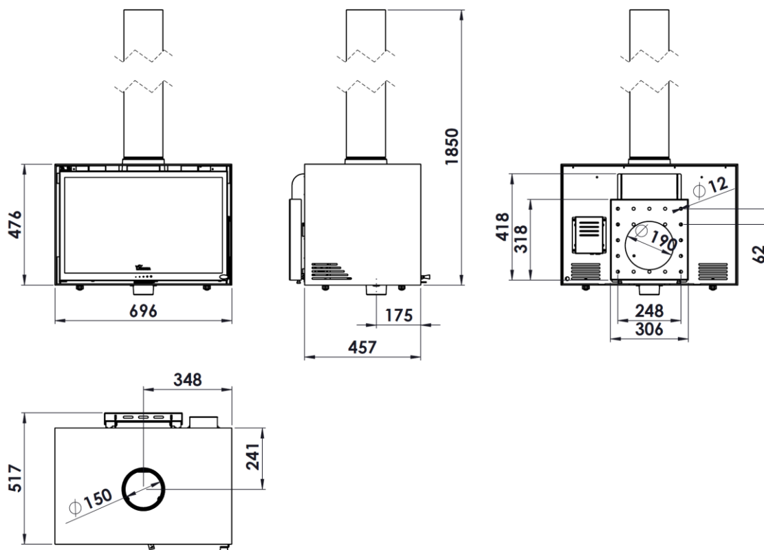
Figura nº2 - Dimensiones en mm del aparato BAIONA 700 STAR MURAL
