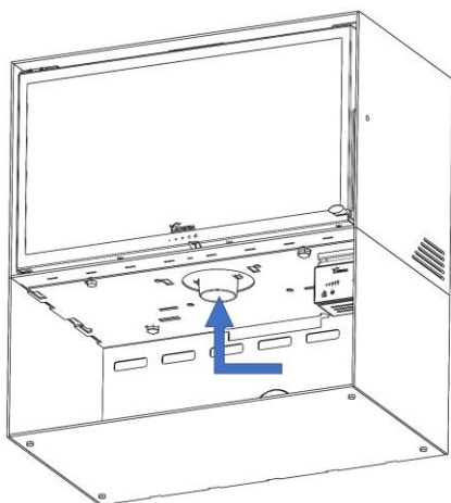
Figura nº8 - Conducción de aire para cámara de combustión
