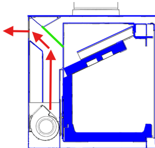
Figura nº18 - Recorrido del aire caliente con canalización
