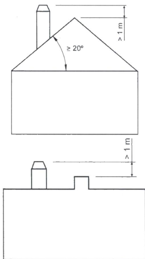
Figura n°19 - Distancias desde el remate hasta la cumbrera del tejado
