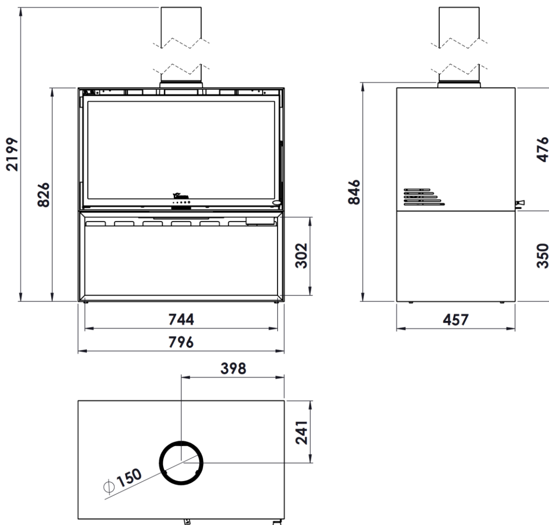
Figura nº3 - Dimensiones en mm del aparato BAIONA 800 STAR
