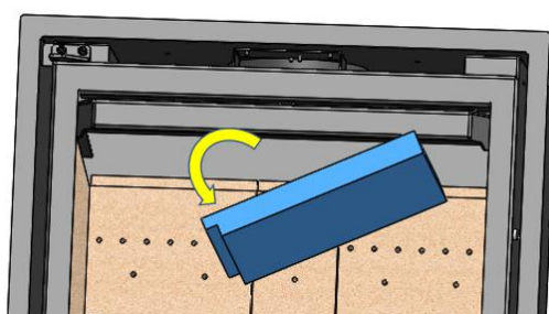
Figura nº26 - Desmontaje de los deflectores inferiores de vermiculita.
