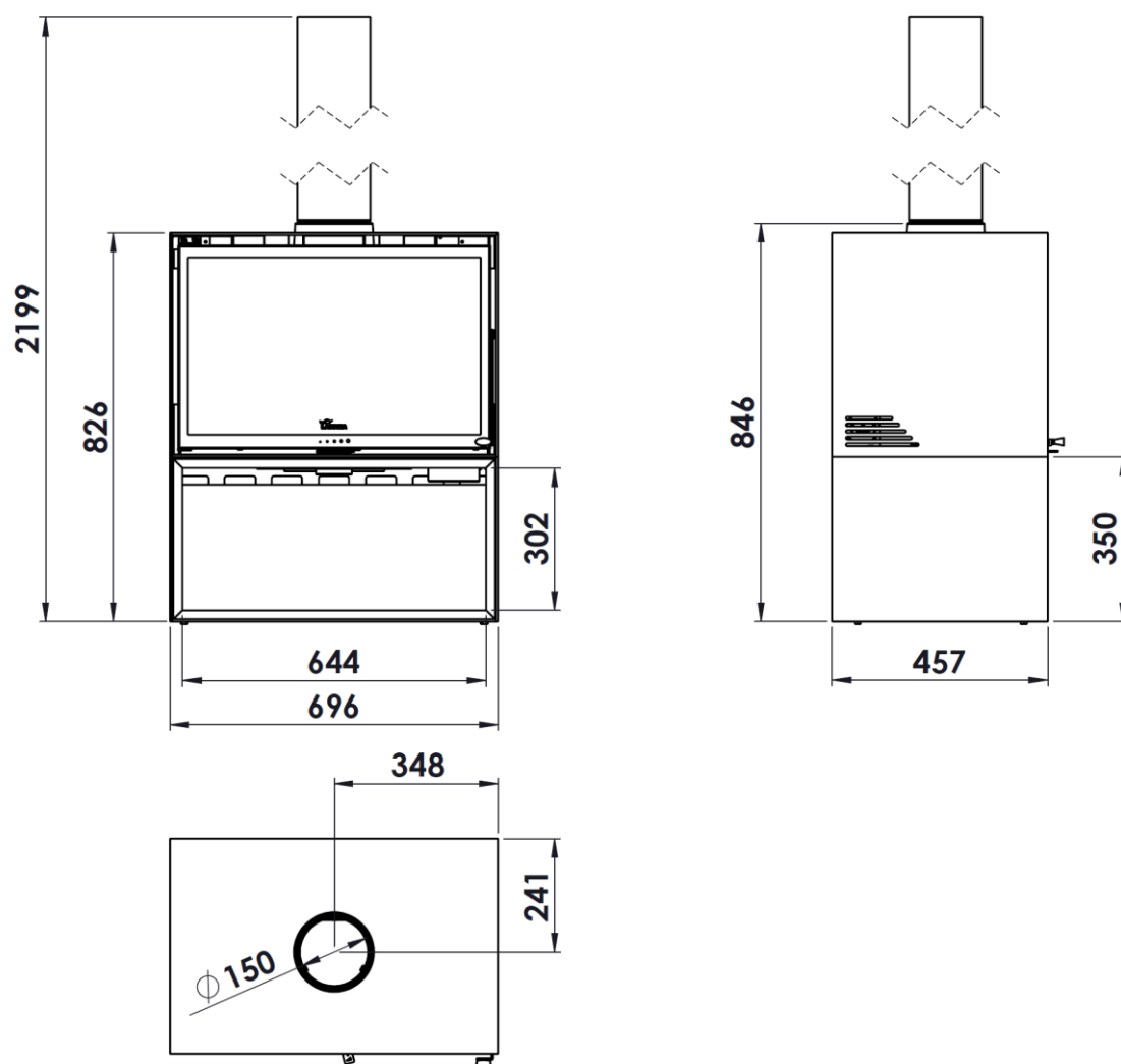
Figura nº1 - Dimensiones en mm del aparato BAIONA 700 STAR
