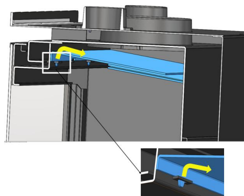
Figura nº27 - Desmontaje del deflector de chapa superior.
