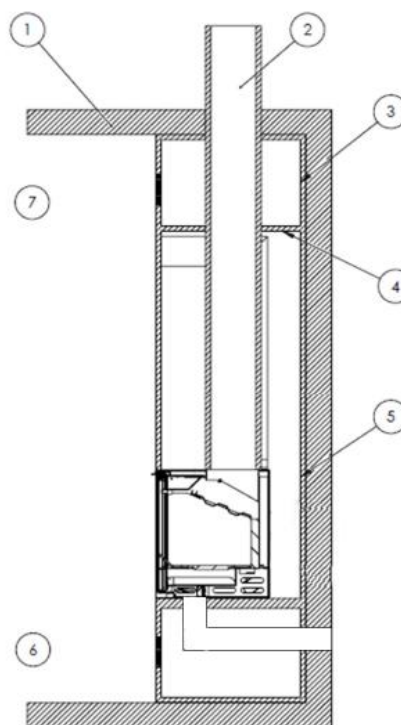
Figura nº7 - Esquema interior del cerramiento
