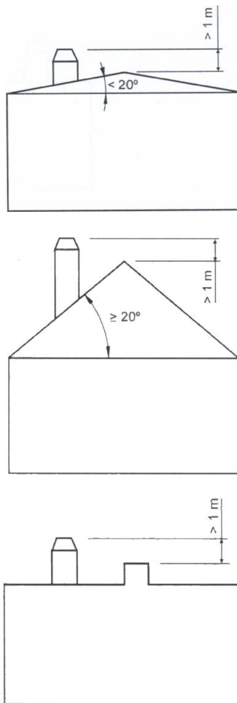
Figura nº19 - Distancias desde el remate hasta la cumbrera del tejado
