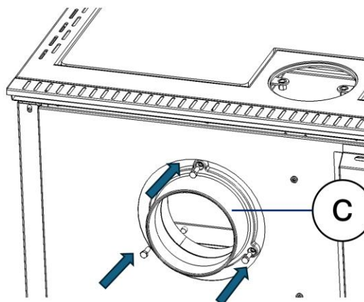
Abbildung 6 - Wir platzieren die hintere Rauchauslässe (C).
