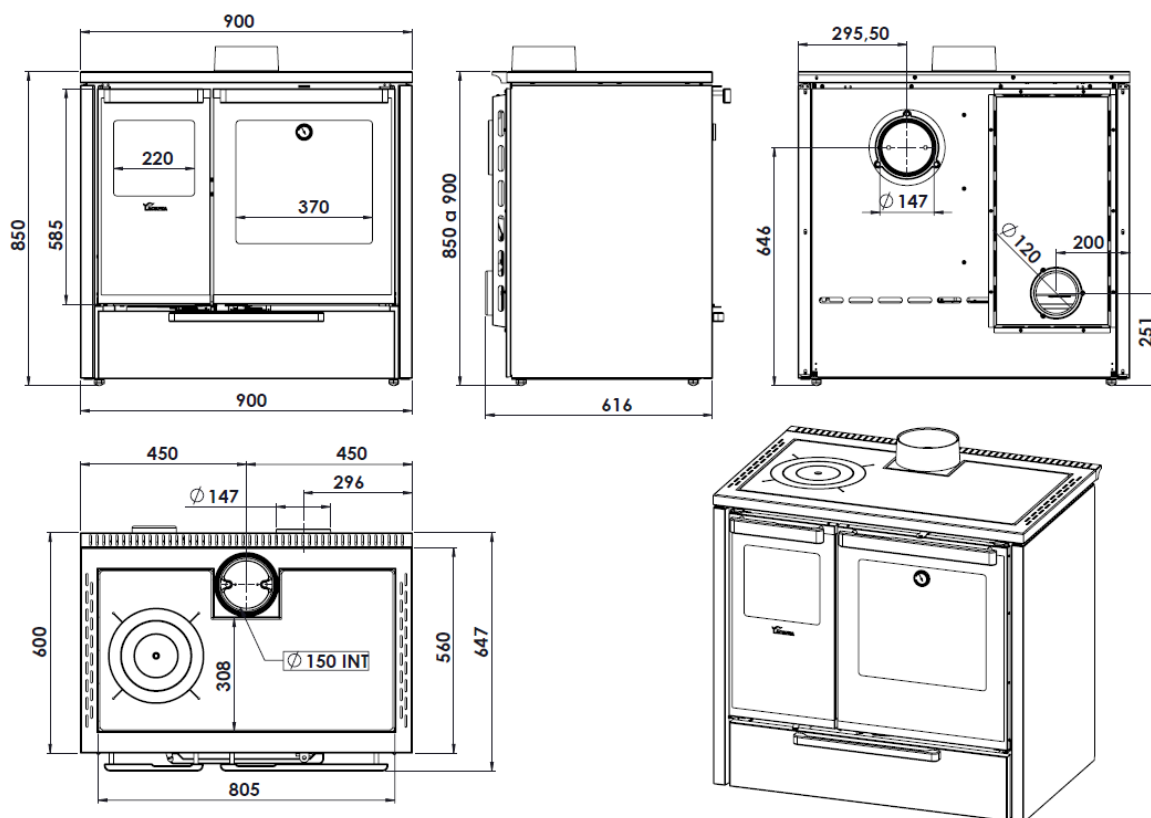
Abbildung Nr. 3 - Abmessungen des Geräts in mm TERRA 7T S-SUP CEN Edelstahl
