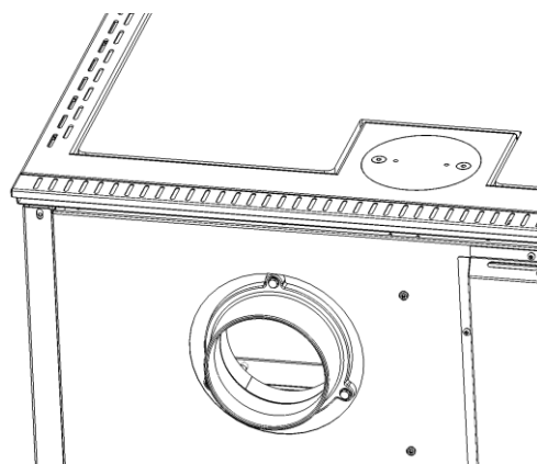
Abbildung Nr. 8 - Endgültiger Ort, geeignet für den hinteren Rauchauslass.
