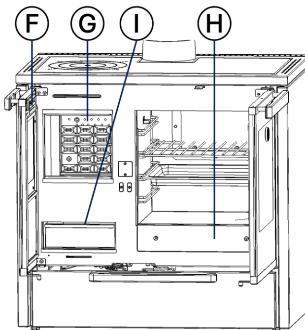
Abbildung Nr.13 - Bedienelemente des Geräts
