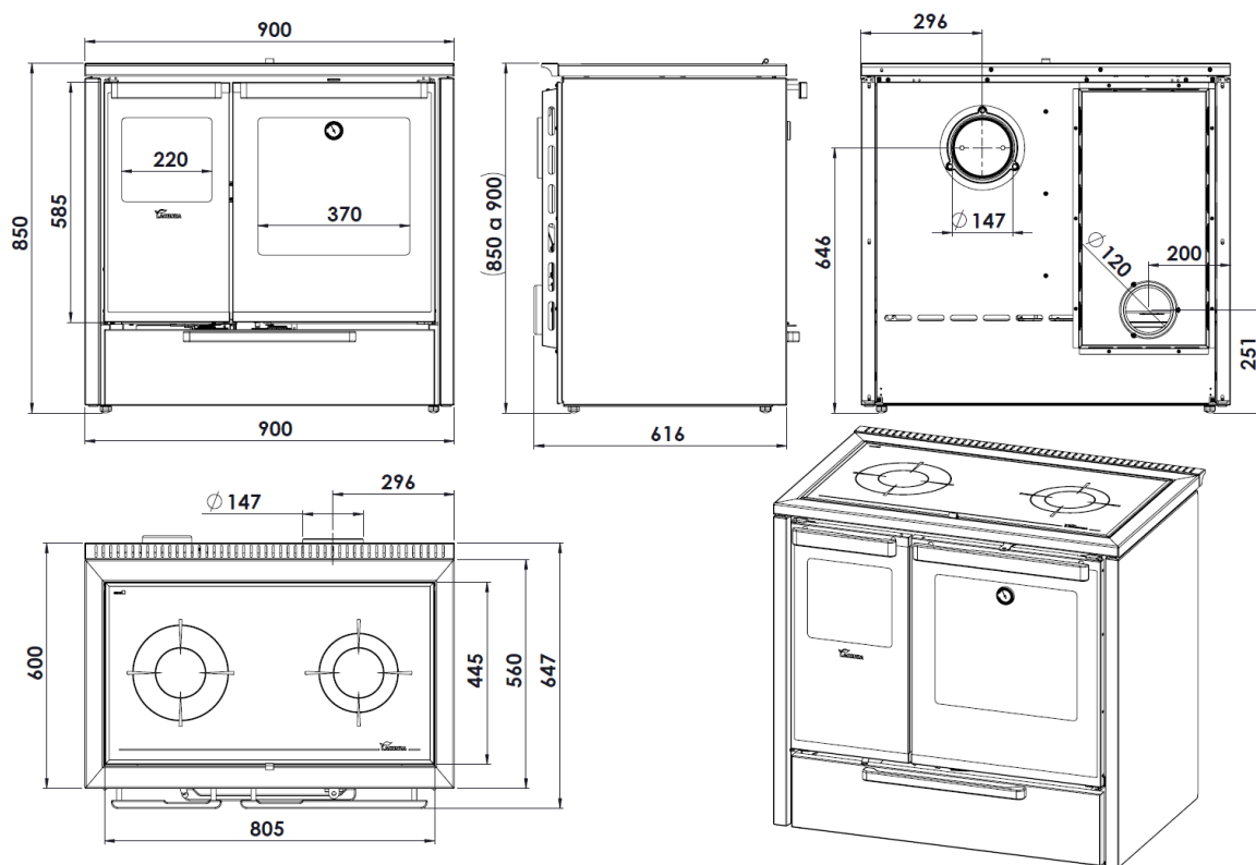
Abbildung Nr.4 - Abmessungen des Geräts in mm TERRA 7T Super V
