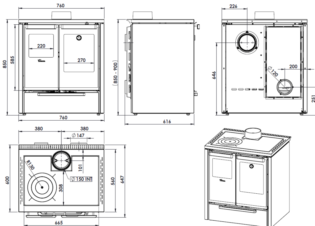
Abbildung Nr.1 - Abmessungen des Geräts in mm TERRA 5T S-SUP CEN Edelstahl
