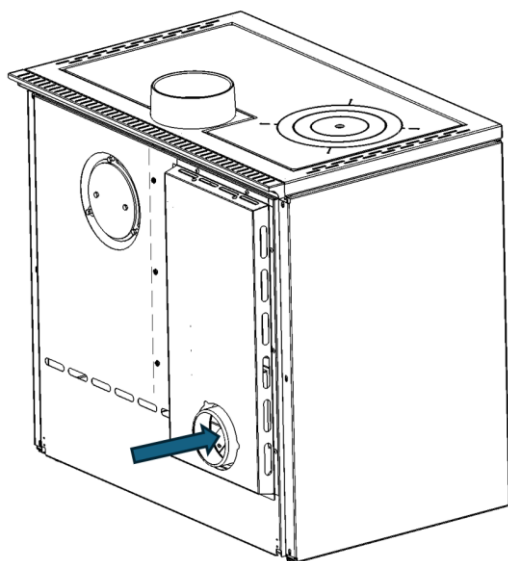
Luftkanal für die Brennkammer
