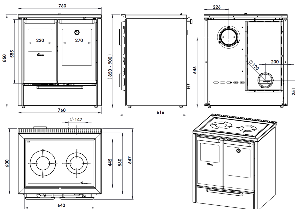
Abbildung Nr. 2 - Abmessungen des Geräts in mm TERRA 5T Super V
