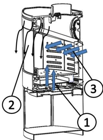
Abbildung Nr.16- Verbrennungslufteinlässe
