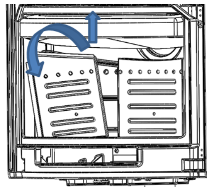
e- Entfernen Sie das Vermiculit (7)
