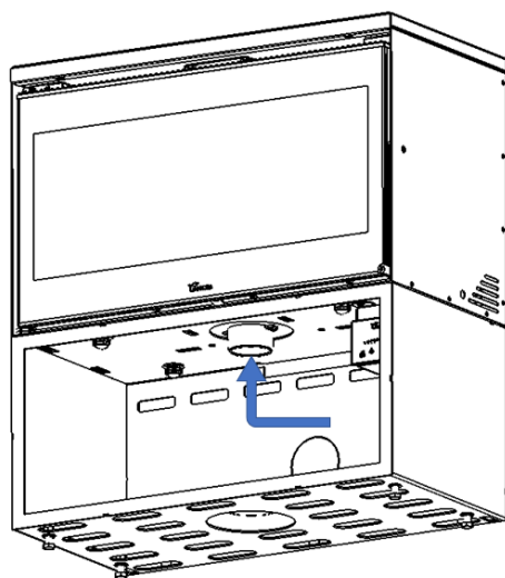
Figura n°9 - Luftführung für die Brennkammer
