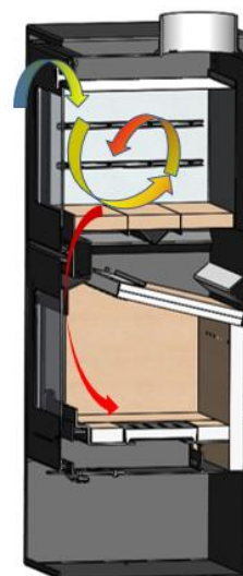
Abbildung 1 - Schema des Rauchabzugsystems
