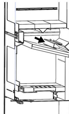
Abbildung Nr. 1 - Verstärkung auf den Vermiculit-Deflektoren
