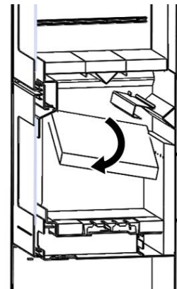
Abbildung 1 - Entfernung von Vermiculit-Prallblechen
