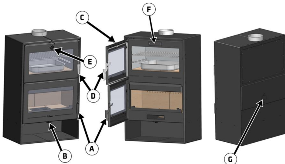
Abbildung 1 - Bedienungselemente des Geräts
