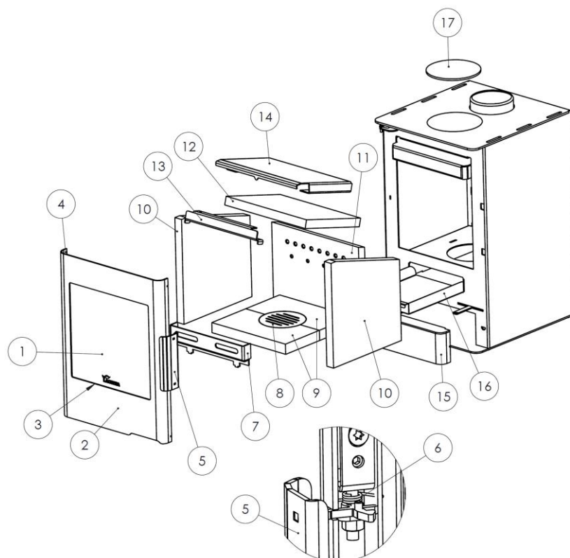
Abbildung Nr.19 – NOMAD Explosionszeichnung
