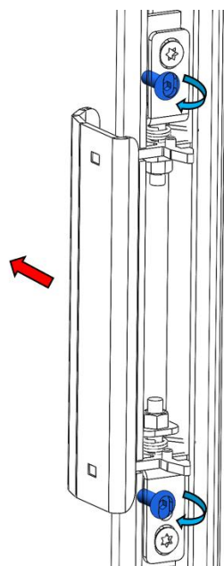
Abbildung Nr.17 - SCHRITT 2: Ziehe die Schrauben fest, die die Tiefe auf die gewünschte Stelle regeln
