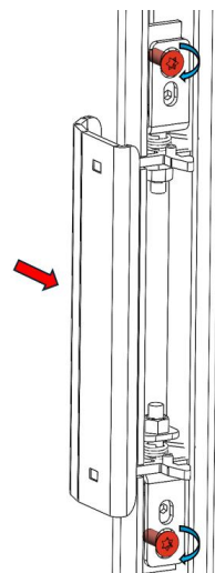
Abbildung Nr.15 - SCHRITT 3: Schrauben festziehen, um das System wieder anzubringen
