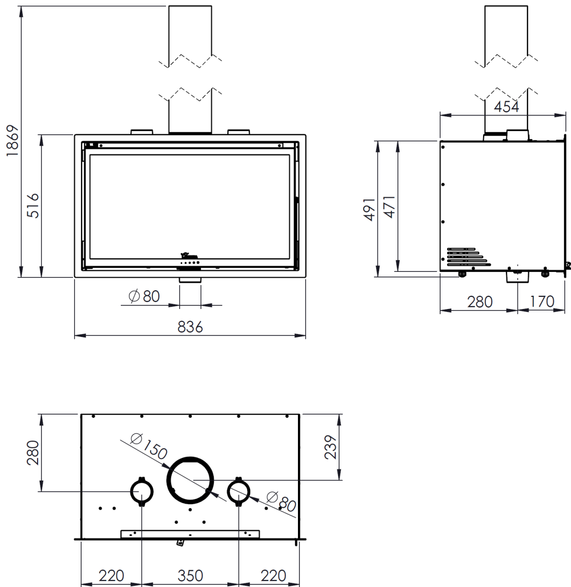
Figura n°2 - Abmessungen in mm del Produkts NIVE 800
