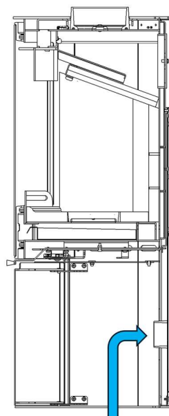
Abbildung Nr.8- OPTION 3 Luftkanal für die Brennkammer
