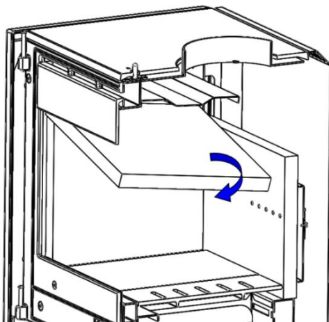
Figura n°2 - Entfernen der Vermiculit-Schallwandteile
