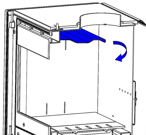
Figura n°4 - Demontage des Stahlabweisers
