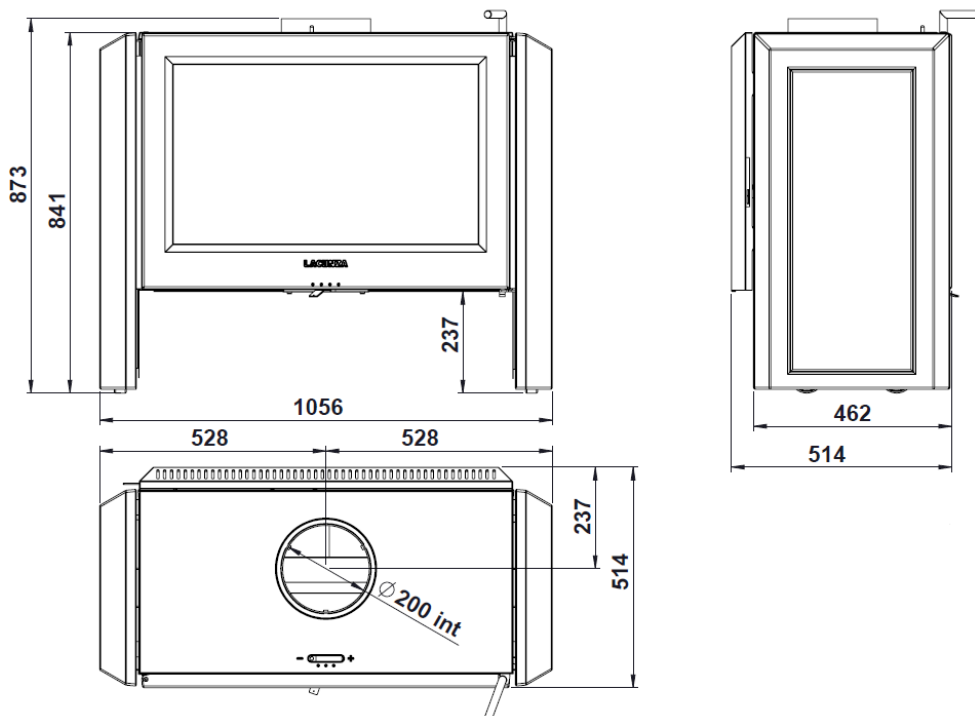
Abbildung 1 Abmessungen des Geräts in mm LEON
