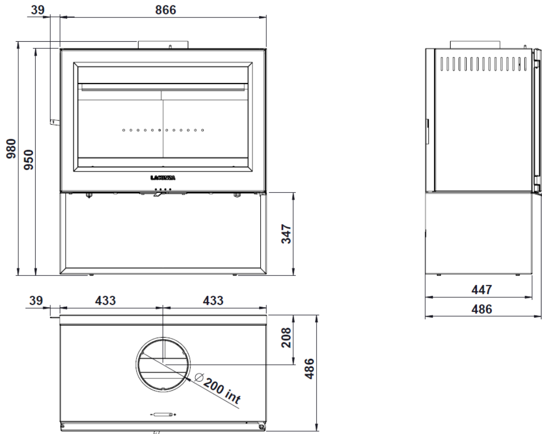
Abbildung 2 Abmessungen des Geräts in mm LUGO
