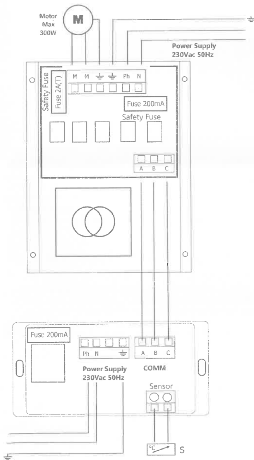
Figura nº8 - Anschlüsse am Steuergerät und Leistungsmodul des Itaca Eco C/V
