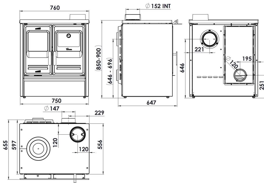
Abbildung Nr.1 - Abmessungen des Geräts in mm ETNA 5T AUSGANG OBEN UND HINTEN
