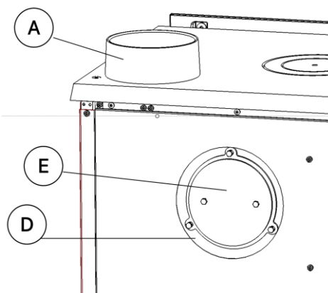
Abbildung Nr. 8 - Endsituation, geeignet für den oberen Rauchabzug.
