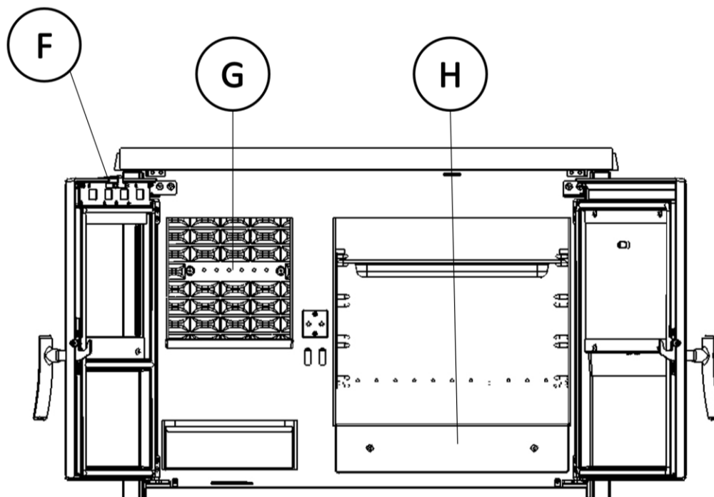
Abbildung Nr.13 - Bedienungselemente des Geräts
