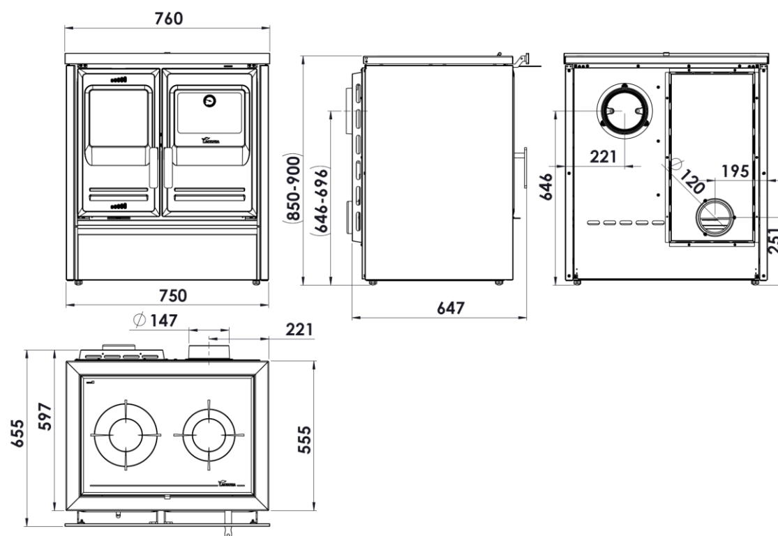
Abbildung Nr. 2 - Abmessungen des Geräts in mm ETNA 5T TOP
