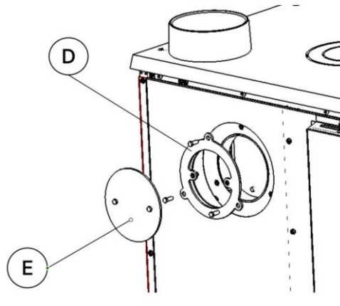
Abbildung Nr. 7 - Montieren Sie den Adapter und die Abdeckung.
