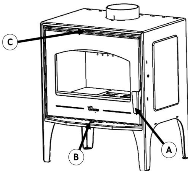
Abbildung 2 Bedienungselemente des Geräts
