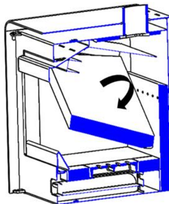
Abbildung 4 Entfernen der Vermiculit-Schikanen
