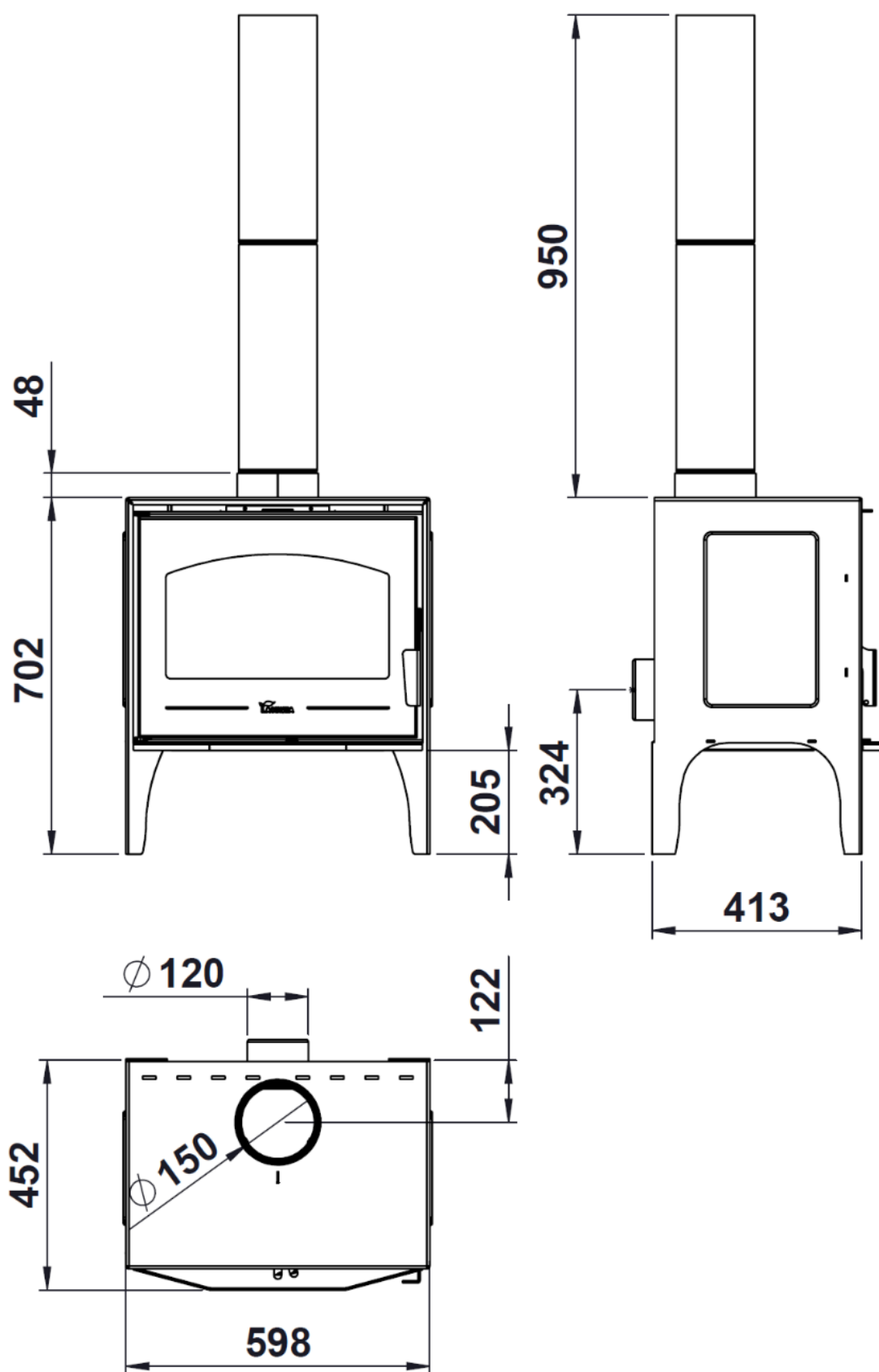
Abbildung 1 Abmessungen des Geräts in mm Calpe
