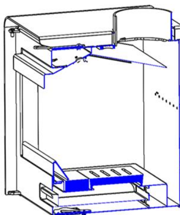
Abbildung 5 Entfernen der restlichen Vermiculite
