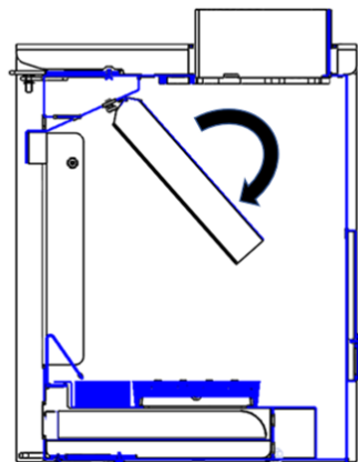
Abbildung 6 Drehen und Entfernen des oberen Stahlabweisers
