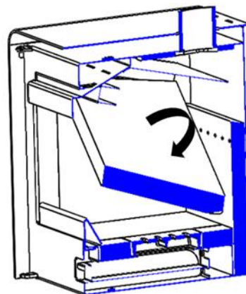
Abbildung 4 Entfernen der Vermiculit-Schikanen
