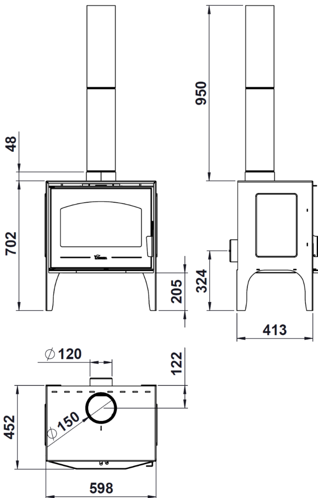
Abbildung 1 Abmessungen des Geräts in mm CALPE STAR
