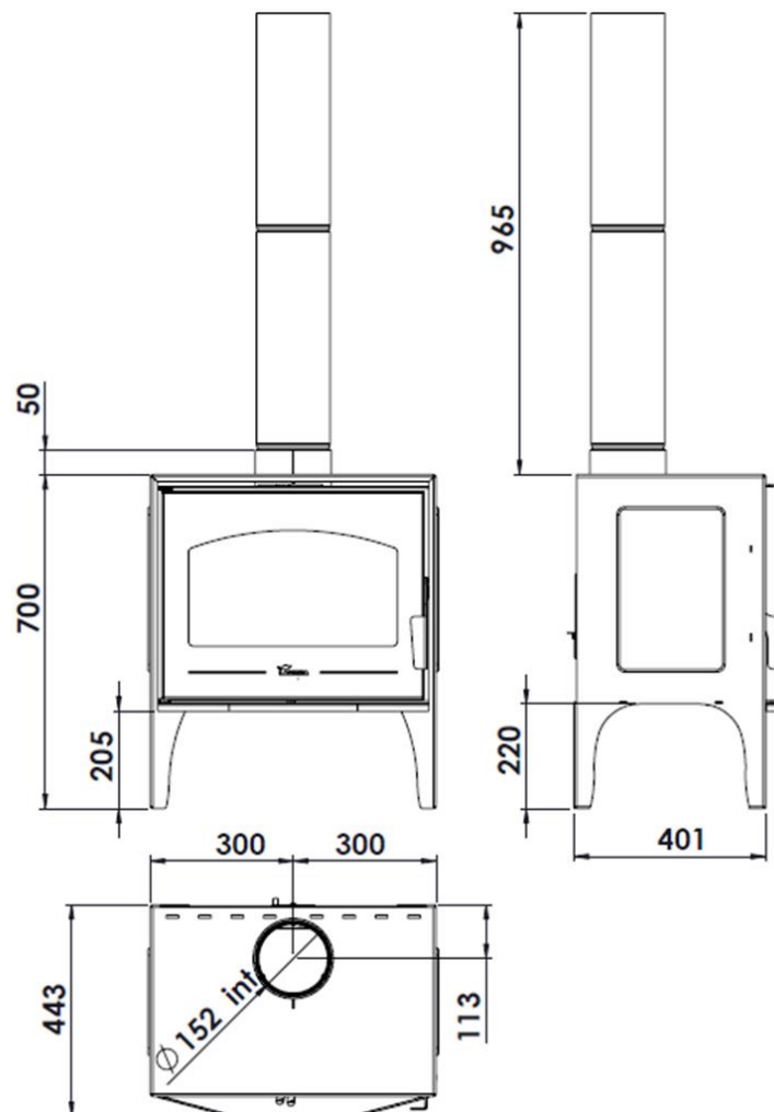
Abbildung 1 Abmessungen des Geräts in mm CALPE
