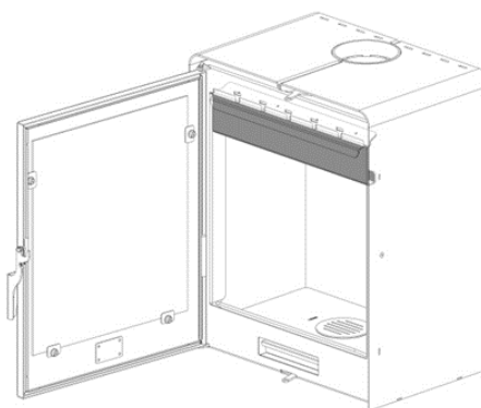
Abbildung 6 Zubehör zur Hilfe in Fällen von Rauchverputz, der durch schlechte Installation verursacht wurde
