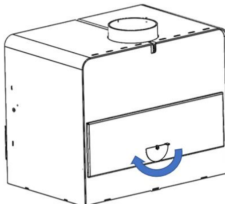
Abbildung 10 Verbrennungslufteinlassregister geschlossen
