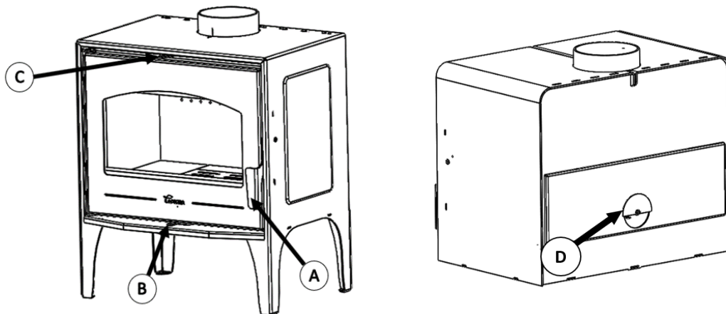
Abbildung 8 Bedienungselemente des Geräts
