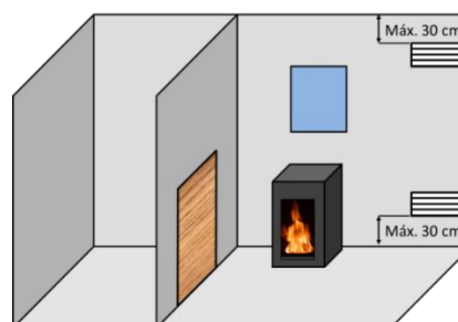
Abbildung 2 Ausrichtungsdiagramm für Lüftungsgitter
