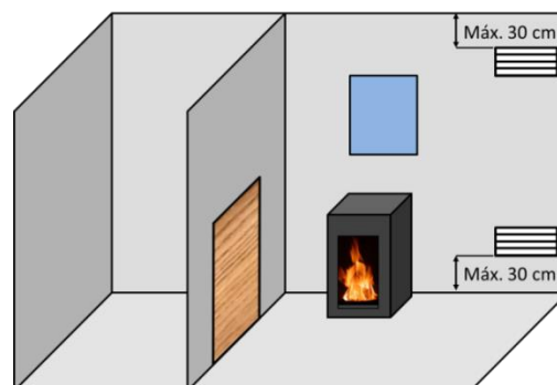
Abbildung 3 Ausrichtungsdiagramm für Lüftungsgitter
