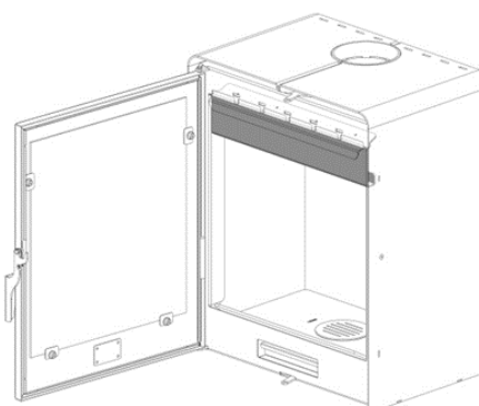
Abbildung 7 Zubehör zur Hilfe in Fällen von Rauchverputz, der durch schlechte Installation verursacht wurde
