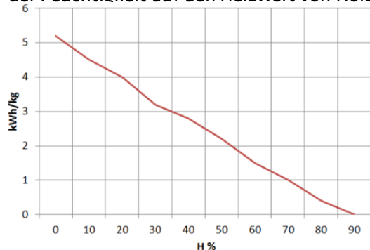
Abbildung 8 Beziehung zwischen Feuchtigkeit und Heizwert von Holz
