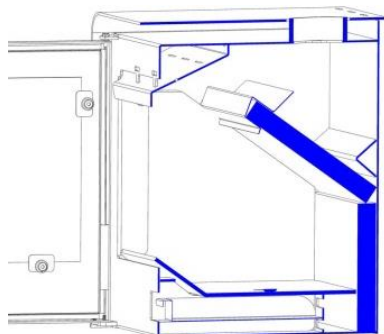
Abbildung 16 Edelstahlverstärkung in geöffneter Position
