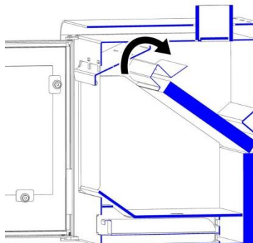
Abbildung 15 Bewegungen, um von der geschlossenen in die offene Position zu gelangen
