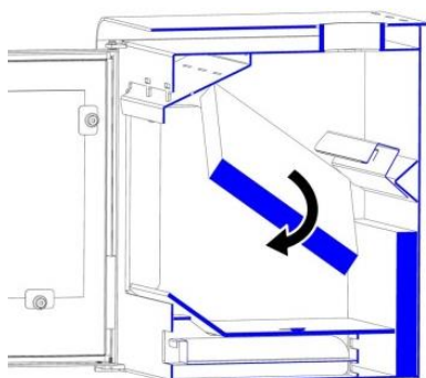
Abbildung 13 Entfernen der Vermiculit-Schikanen
