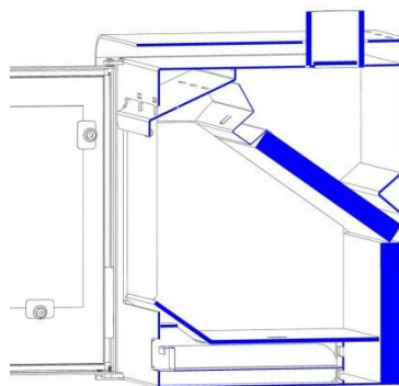
Abbildung 14 Edelstahlverstärkung in geschlossener Position
