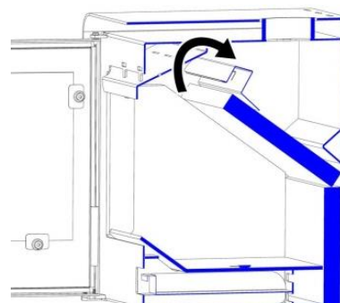
Abbildung 11 Verdrehung der Verstärkung aus rostfreiem Stahl
