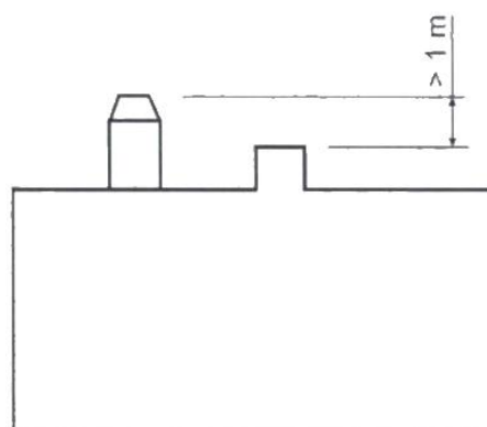
Abbildung 4 Abstände von der Kappe zum Dachfirst
