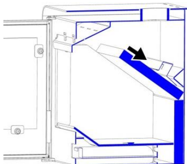
Abbildung 12 Bewehrung an Vermiculit-Schallwänden
