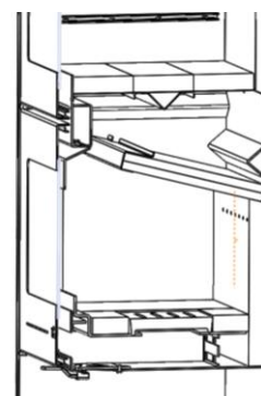
Abbildung 1 - Edelstahlverstärkung in der offenen Position
