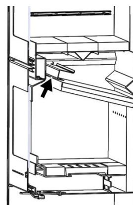
Abbildung n°1 - Drehung der Edelstahlbewehrung
