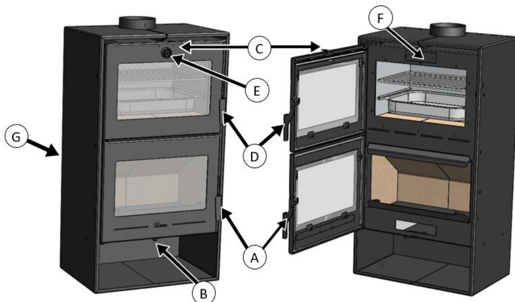
Abbildung 1 - Bedienungselemente des Geräts
