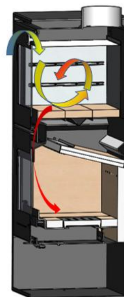
Abbildung 1 - Schema des Rauchabzugssystems
