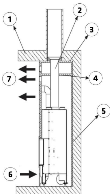
Figura nº3 - Esquema interior del cerramiento
