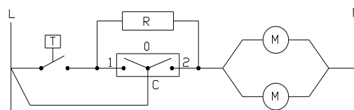
Figura nº11 - Esquema eléctrico de los ventiladores
