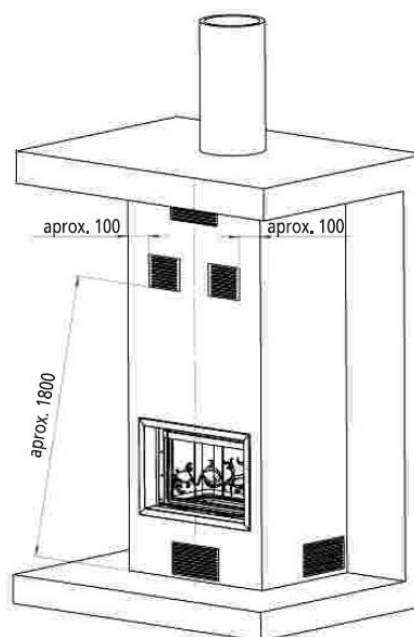
Figura nº4 - Esquema exterior del cerramiento
