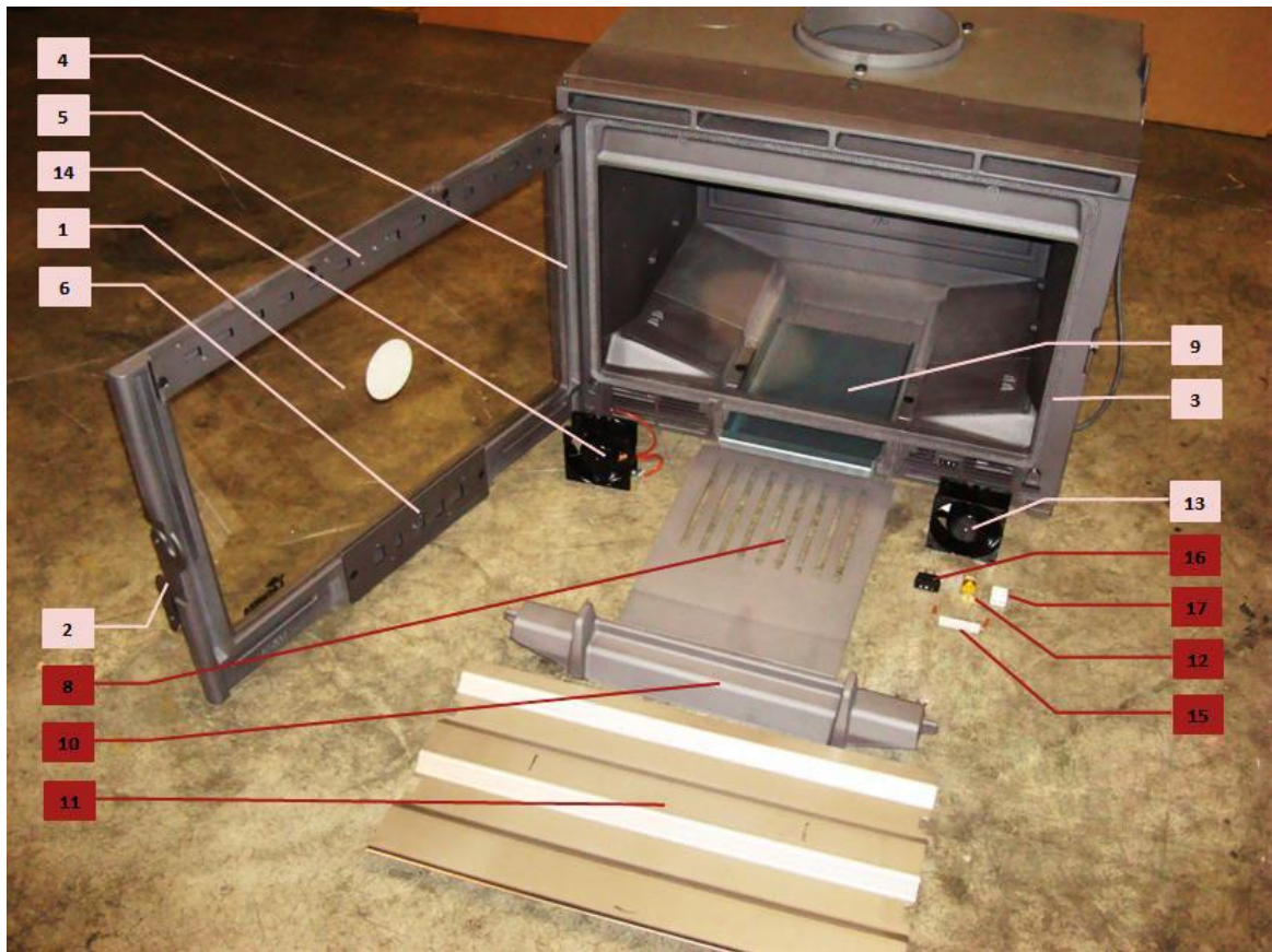
Figura nº12 - Despiece MIDI-700
