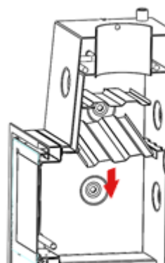
Figura nº17 - Desmontagem do defletor inferior Sarria Plus
