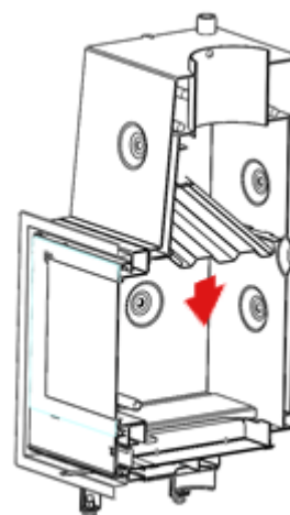
Figura nº15 - Desmontagem do defletor Otazu
