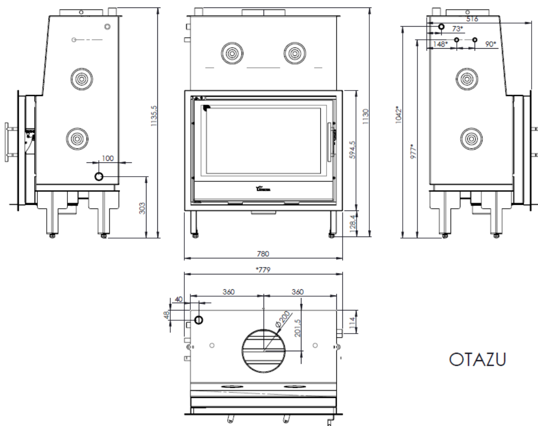
Figura nº1 - Dimensões em mm do aparelho Otazu
