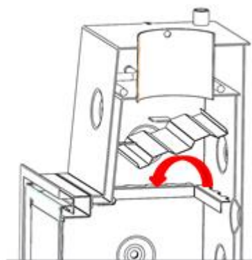
Figura nº18 - Desmontagem do defletor superior Sarria Plus
