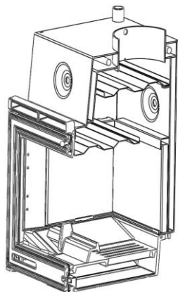
Figura nº19 - Vista de secção com dois defletores instalados (Sarría Plus)
