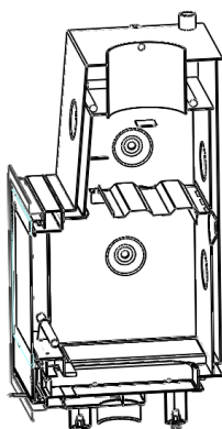
Figura nº16 - Vista de secção com um defletor instalado (Otazu)
