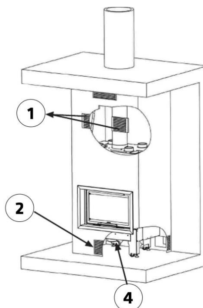
Figura n°8 - Immagine descrittiva dell'opzione A
