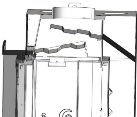
Figura n°19 - Vista in sezione con i 2 deflettori collocati
