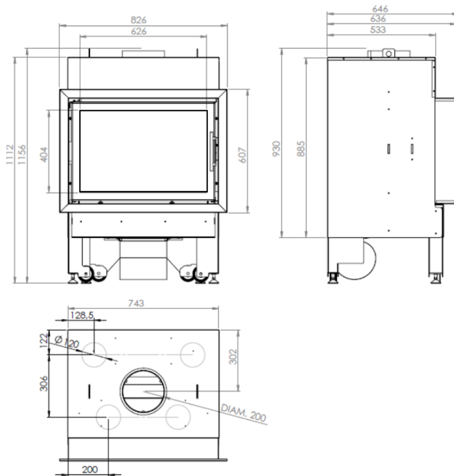
Figura n°1 - Dimensioni in mm dell'apparecchio INCA 80
