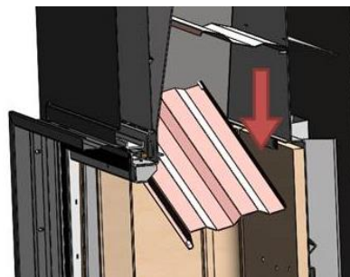
Figura n°21 - Smontaggio del deflettore inferiore Inca
