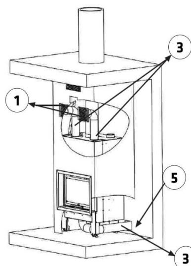
Figura n°11 - Immagine descrittiva dell'opzione D
