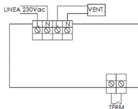
Figura n°13 - Collegamenti da realizzare nel potenziometro della turbina inca
