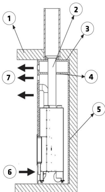
Figura n°5 - Schema interno del rivestimento
