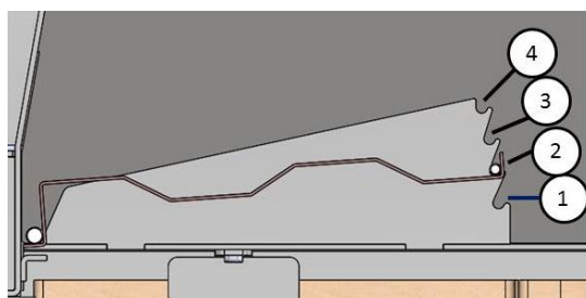
Figura n°20 - Diverse posizioni del deflettore inferiore Inca
