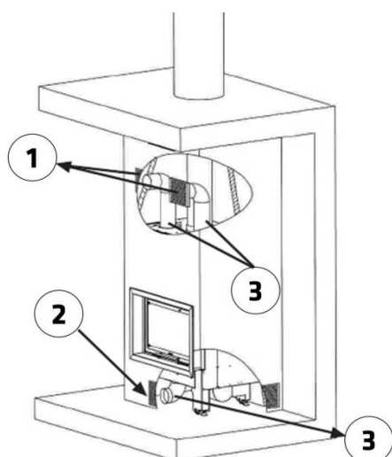
Figura n°9 - Immagine descrittiva dell'opzione B
