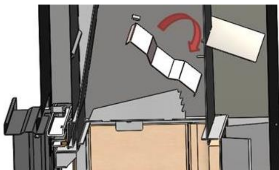
Figura nº22 - Smontaggio del deflettore intermedio Inca
