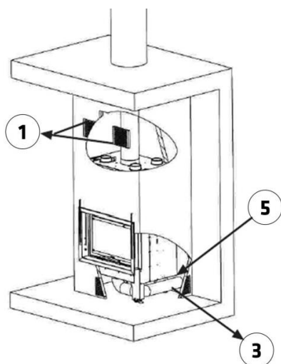
Figura n°10 - Immagine descrittiva dell'opzione C
