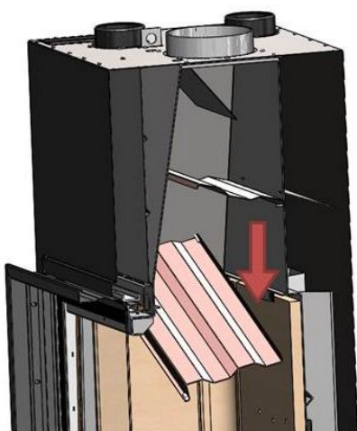
Figura nº24 - Desmontaje del deflector inferior Itaca
