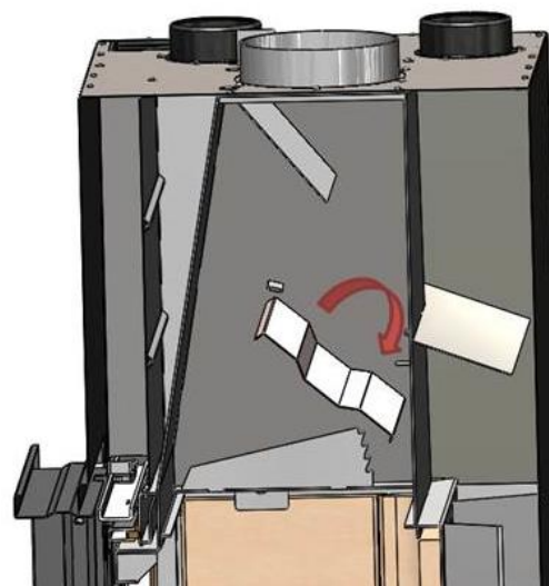
Figura nº25 - Desmontaje del deflector medio Itaca
