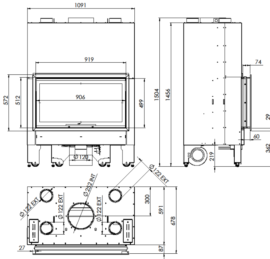
Figura n o 2 - Dimensiones en mm aparato Itaca 100
