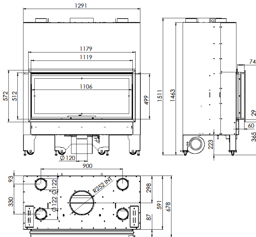
Figura n o 3 - Dimensiones en mm Itaca 120
