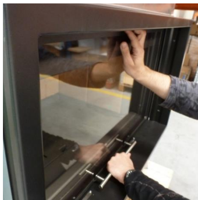
Figura nº30 - Sujetar el tirador con una de las manos mientras que con la otra tiramos de la puerta hacia fuera.
