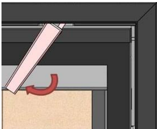
Figura nº29 - Girar el pivote dcho en el sentido de agujas reloj
