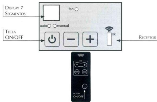
Figura nº35 - Display potenciómetro Itaca
