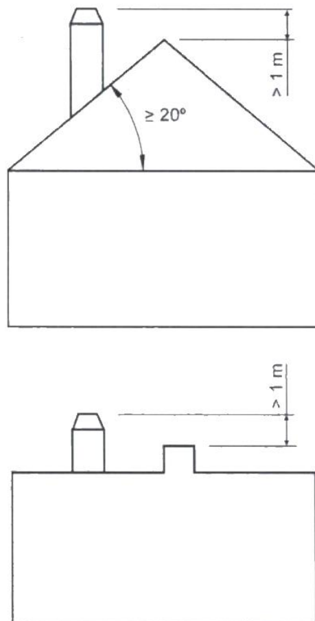
Figura nº17 - Distancias desde el remate hasta la cumbrera del tejado
