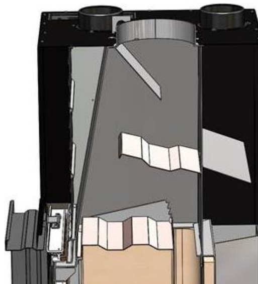
Figura nº22 - Vista de sección con los 3 deflectores colocados
