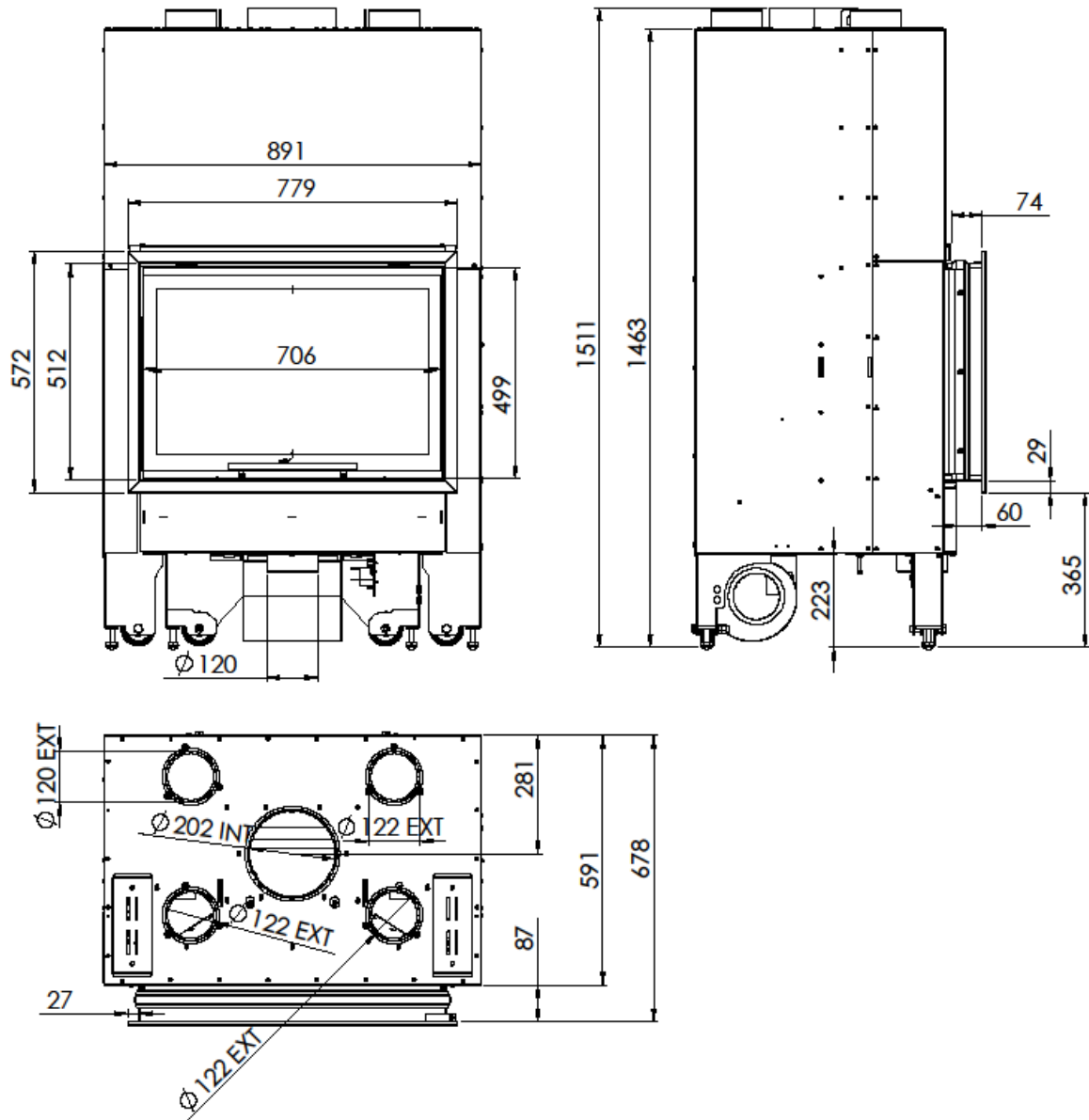
Figura nº1 - Dimensiones en mm del aparato ITACA 80
