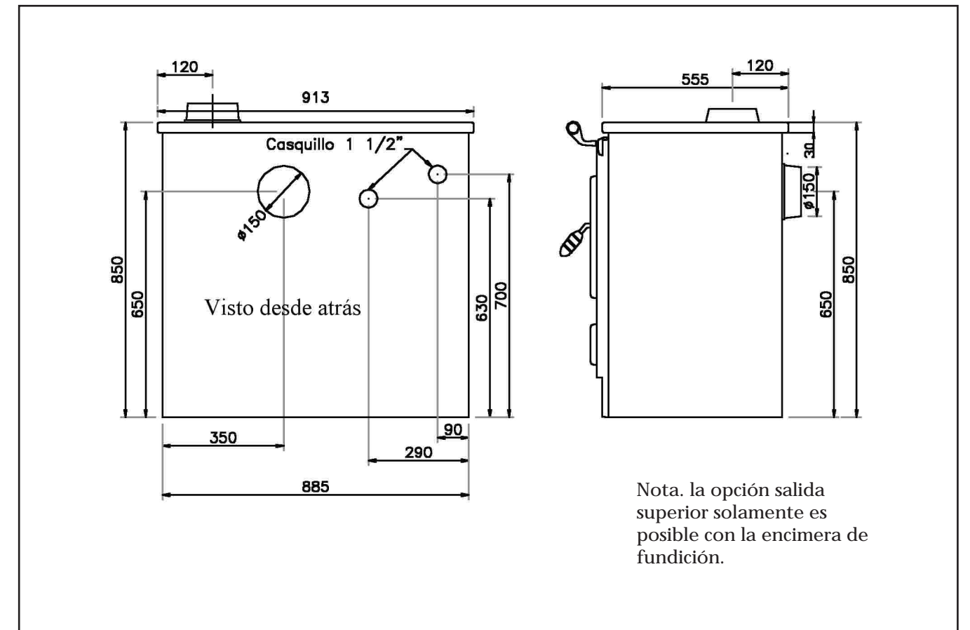
Figura n° 1 - Dimensiones en mm. Cocina Lis 5TE.
